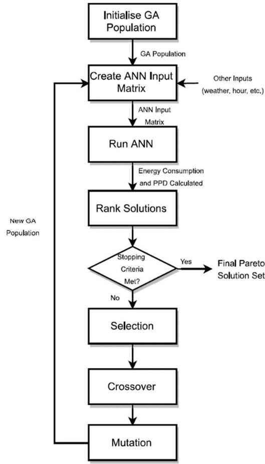
Fig. 4. Optimisation Procedure
